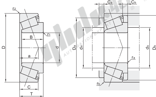
安装图
