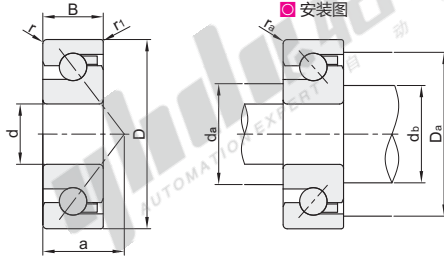
安装图
