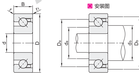
安装图
