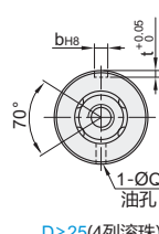
D ≥ 25 (4列滚珠)
