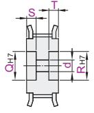
Y 两端台阶孔
