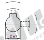
N 新JIS键槽+螺孔 C 旧JIS键槽+螺孔
