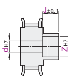
F 台阶孔 (轮毂侧沉孔)
