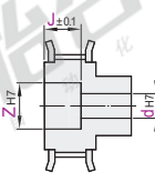
V 台阶孔
