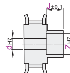
F 台阶孔 (轮毂侧沉孔)
