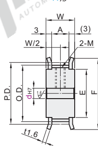
带轮形状 A形
