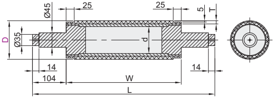
涂布牵引型 QAA76
