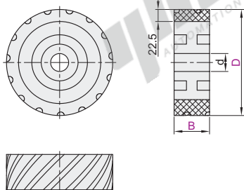
田形:主动轮 QBR71
