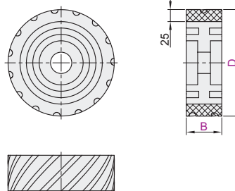
田形:从动轮 QBR72
