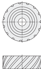
田形:从动轮 QBR76
