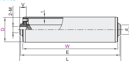
内螺纹型 QCE21/31/32
