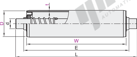
扁位型 QCE41/51/52
