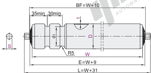
双槽型-弹簧压入式 QCH01 QCH02
