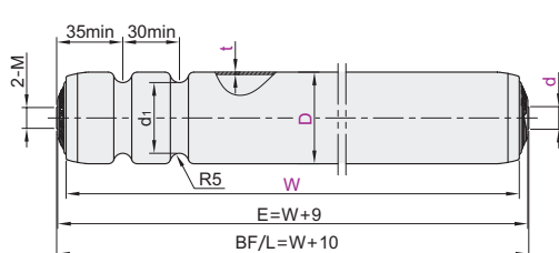
双槽型-内螺纹型 QCH11 QCH12
