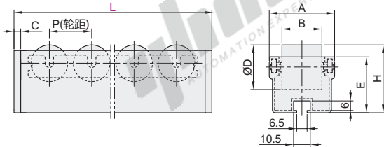
树脂轮型 QJK05
