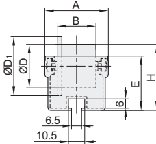
法兰轮型 QJK04
