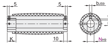
键槽+螺孔型
