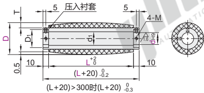
圆孔+螺孔型
