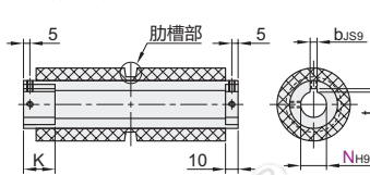
键槽+螺孔型
