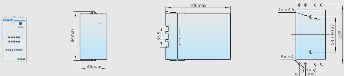
XJ3-G外形及安装尺寸
