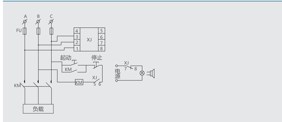
XJ3-G接线图
