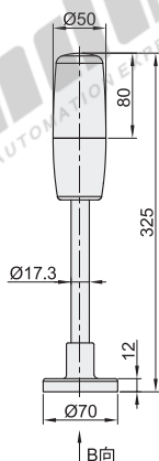
C(杆盘式)
