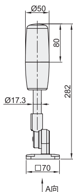
A(可折式)
