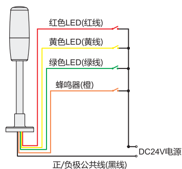
接线图
