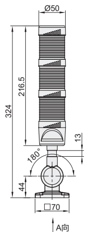
A(可折式)
