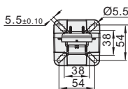
A向视图
