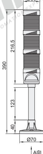
C(杆盘式)
