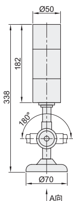
A(可折式)
