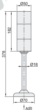
C(杆盘式)
