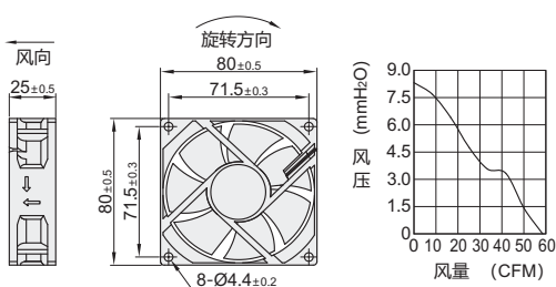
外形尺寸: 8025M1
