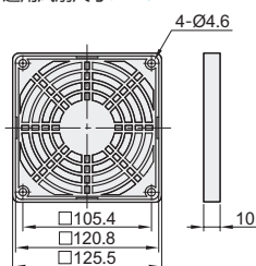
铁网
