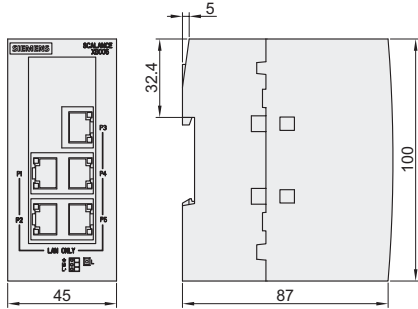
端口数:5 6GK5005-0GA10-1AB2
