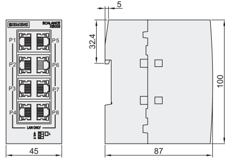
端口数:8 6GK5008-0GA10-1AB2
