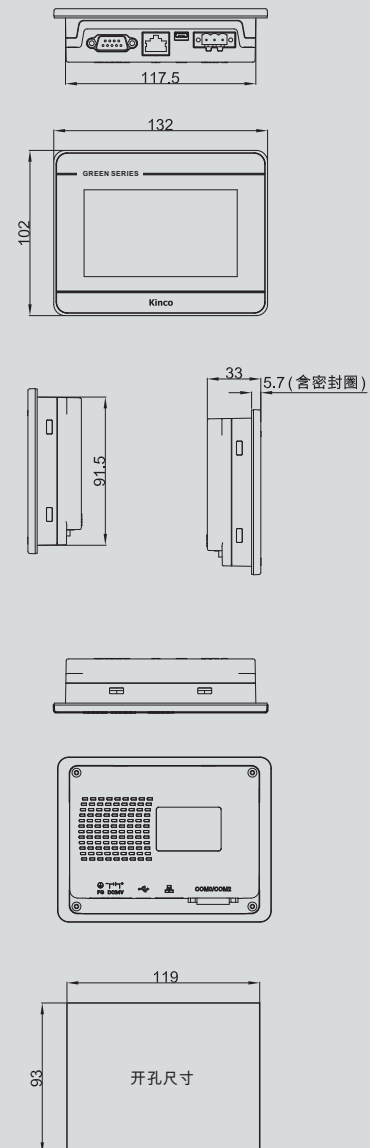
尺寸图 (单位: mm)
