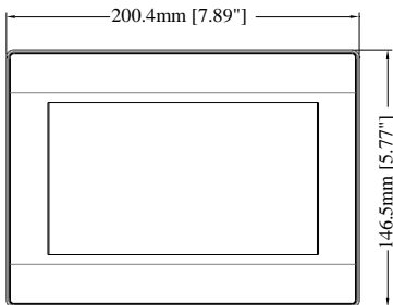
正视图
