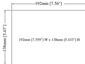
开孔尺寸图
