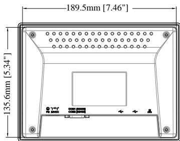
背视图
