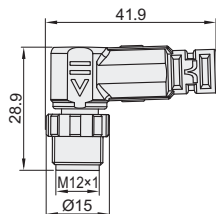
弯公头
