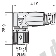
弯母头
