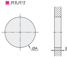
开孔尺寸
