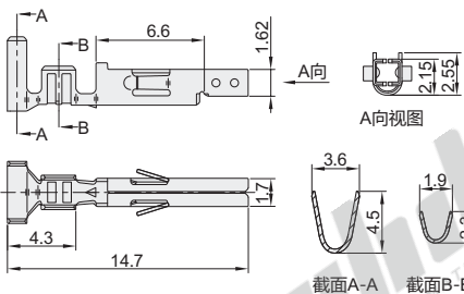
5556系列-端头 39-00-0038
