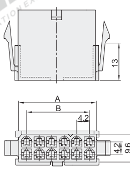
5559系列-公胶壳
