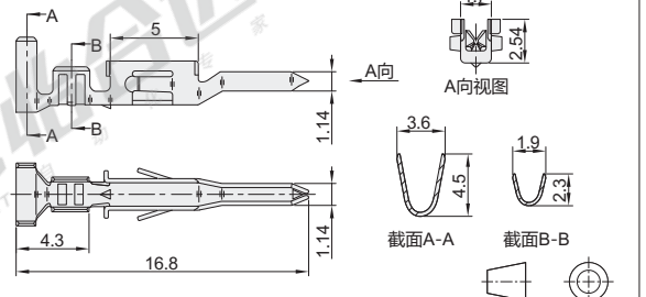
5558系列-端头 39-00-0040
