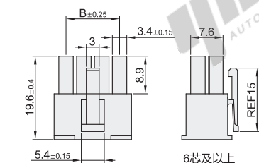
双行公胶壳 ZKY11-M
