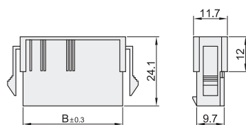
双行母胶壳 ZKY11-F
