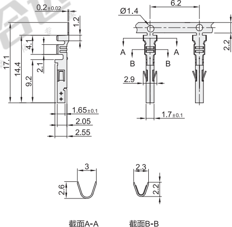
母端头 ZKY12-F
