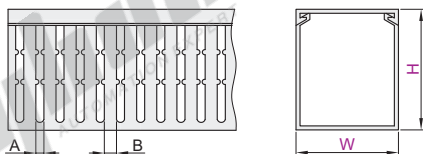
■ W≥80mm线槽底部孔尺寸
