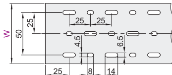
■ W≥80mm线槽底部孔尺寸
