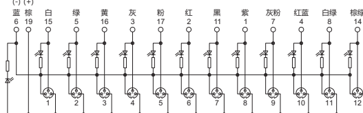
12位 PNP
