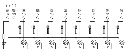
8位 PNP
