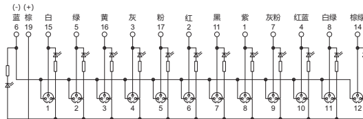
12位 NPN
