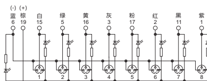
8位 NPN
