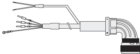
外形图D
