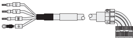
外形图C
