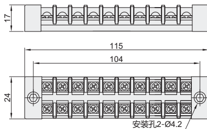
ZIW65-20-15
