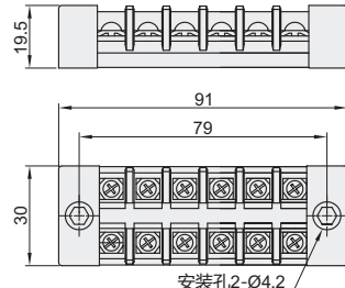
ZIW65-20-6
