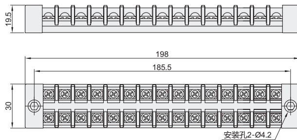
ZIW65-20-15
