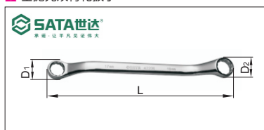
全抛光双梅花扳手
