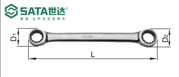
英制全抛光双梅花快扳
