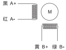
接线图
