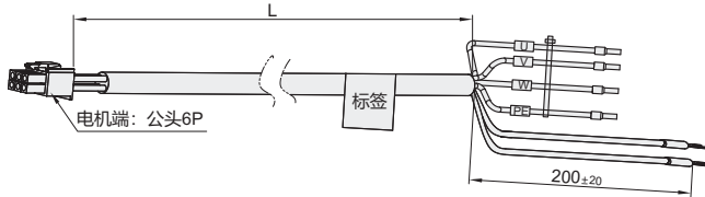
动力刹车线 ZNH32
