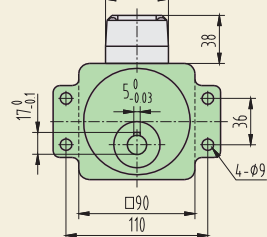
带耳减速箱
