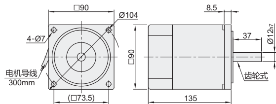
电机 ZKR53
