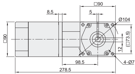
减速机+电机 (输出轴:实心轴) (ZKR53+ZKR13)
