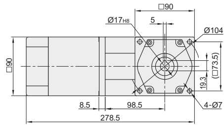
减速机+电机 (输出轴:空心轴) (ZKR53+ZKR14)
