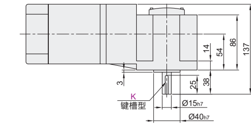
电机 ZKR53
