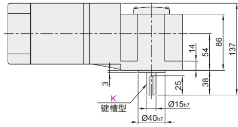
电机 ZKR83
