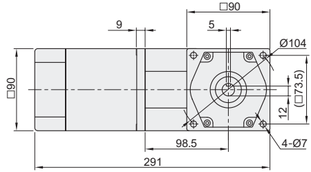
减速机+电机 (输出轴:实心轴) (ZKR83+ZKR13)
