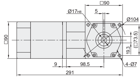
减速机+电机 (输出轴:空心轴) (ZKR83+ZKR14)
