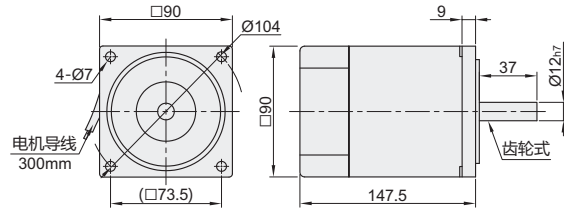
电机 ZKR83
