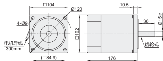
电机 ZKR85
