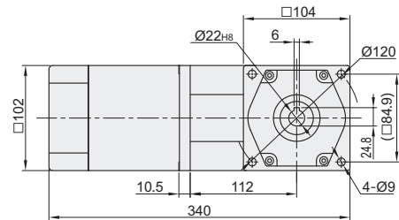
减速机+电机 (输出轴: 空心轴) (ZKR85+ZKR16)
