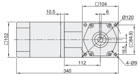
减速机+电机 (输出轴: 实心轴) (ZKR85+ZKR15)
