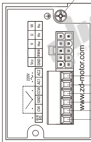
HIGH VOLTAGE DRIVE WIRING 高压驱动接线说明
