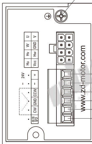
LOW VOLTAGE DRIVE WIRING 低压驱动接线说明
