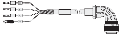
外形图G
