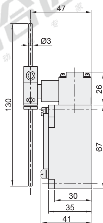
F: 可调圆棒摆杆型
