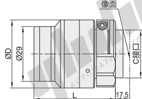
外形图: B
