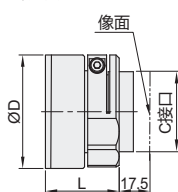
外形图: A
