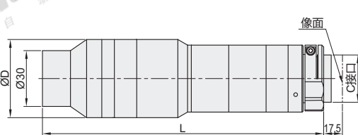
外形图: C
