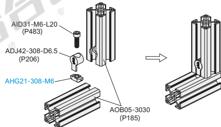
分解图
