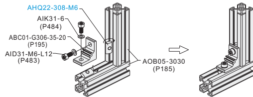
分解图
