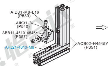
分解图
