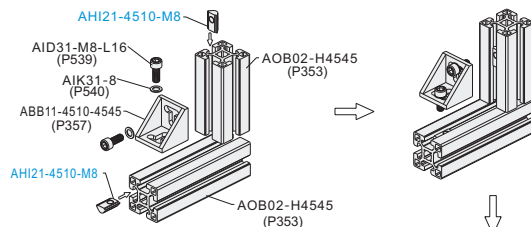
分解图
