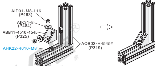
分解图
