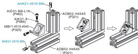
分解图
