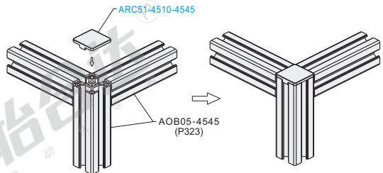
分解图
