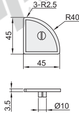
ARC51-4510-4545R ARC52-4510-4545R (只适合怡合达型材)
