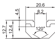
槽口详图
