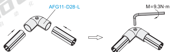
分解图
