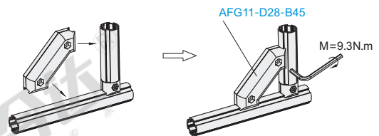
分解图
