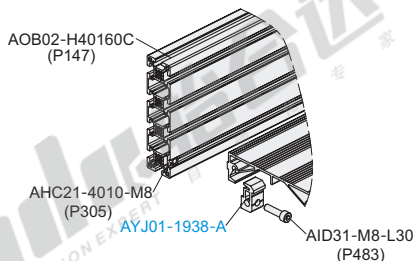
分解图
