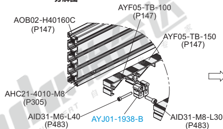
分解图
