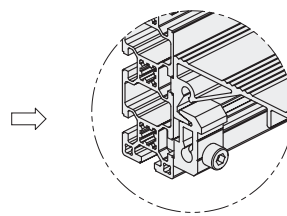
组装图
