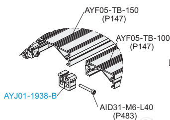
分解图
