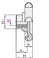
螺孔型
