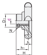
螺钉锁紧型
