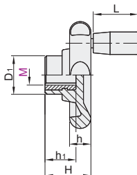
螺孔型
