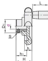
销钉固定型
