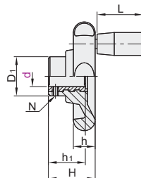
螺钉锁紧型
