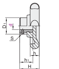
销钉固定型
