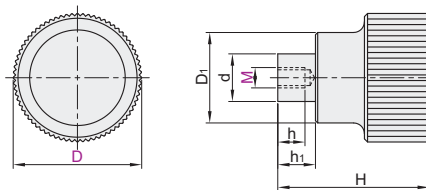
内螺纹型 HAU71
