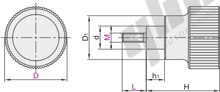
外螺纹型 HAU70
